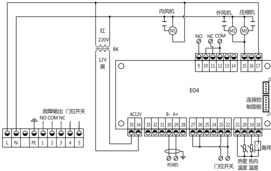
10.3 FCC1100/1500 , 230V AC/50 Hz电路图：
