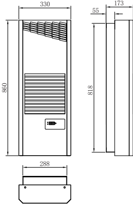
FCC680P/825P外形图和安装开孔图 :
