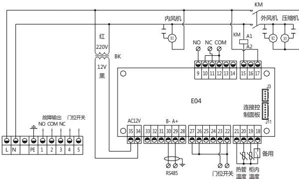
10.3 FCC1100/1500 , 230V AC/50 Hz电路图：
