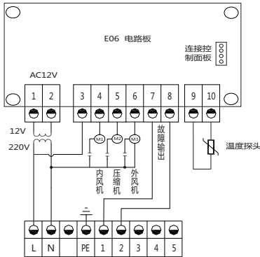
10.1 FCC225/320/ 680/825 , 230V AC/50 Hz电路图：
