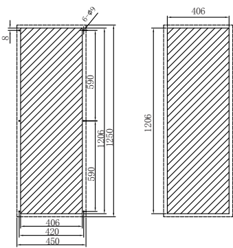
FCC1100/1500安装开孔图： FCC1100Q/1500Q 安装开孔图：
