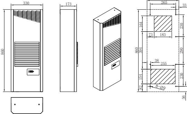
FCC680P/825P外形图和安装开孔图 :
